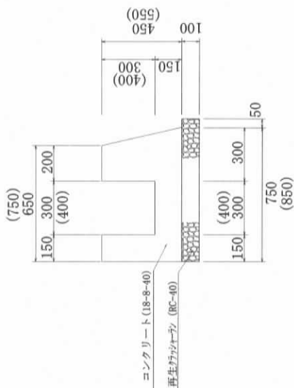
現場打側溝 (B) (G) (U-300×300) (U-400×400)
