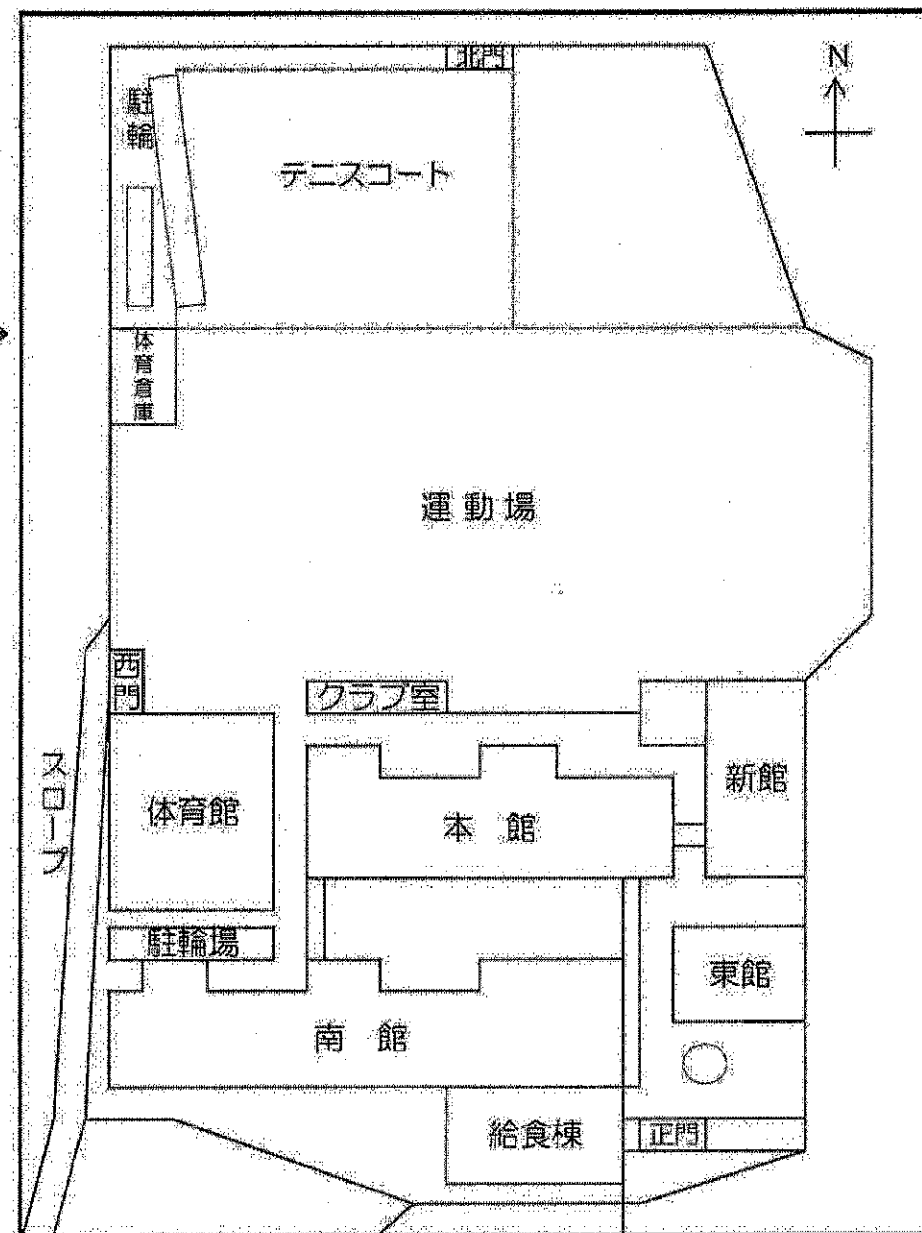
校舎略図・校舎配置図
