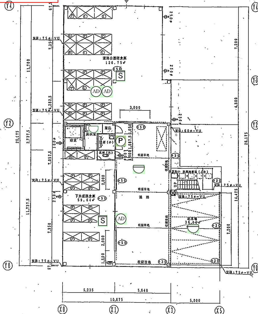
1F 平面図 S1:100
