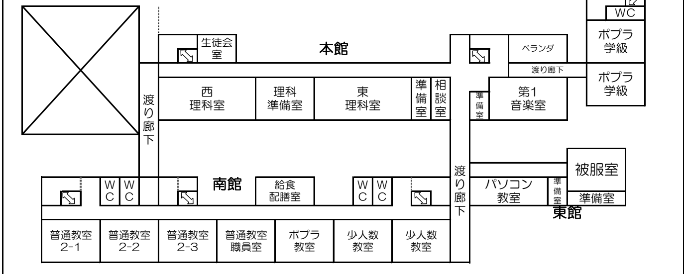
校舎配置図 2F
