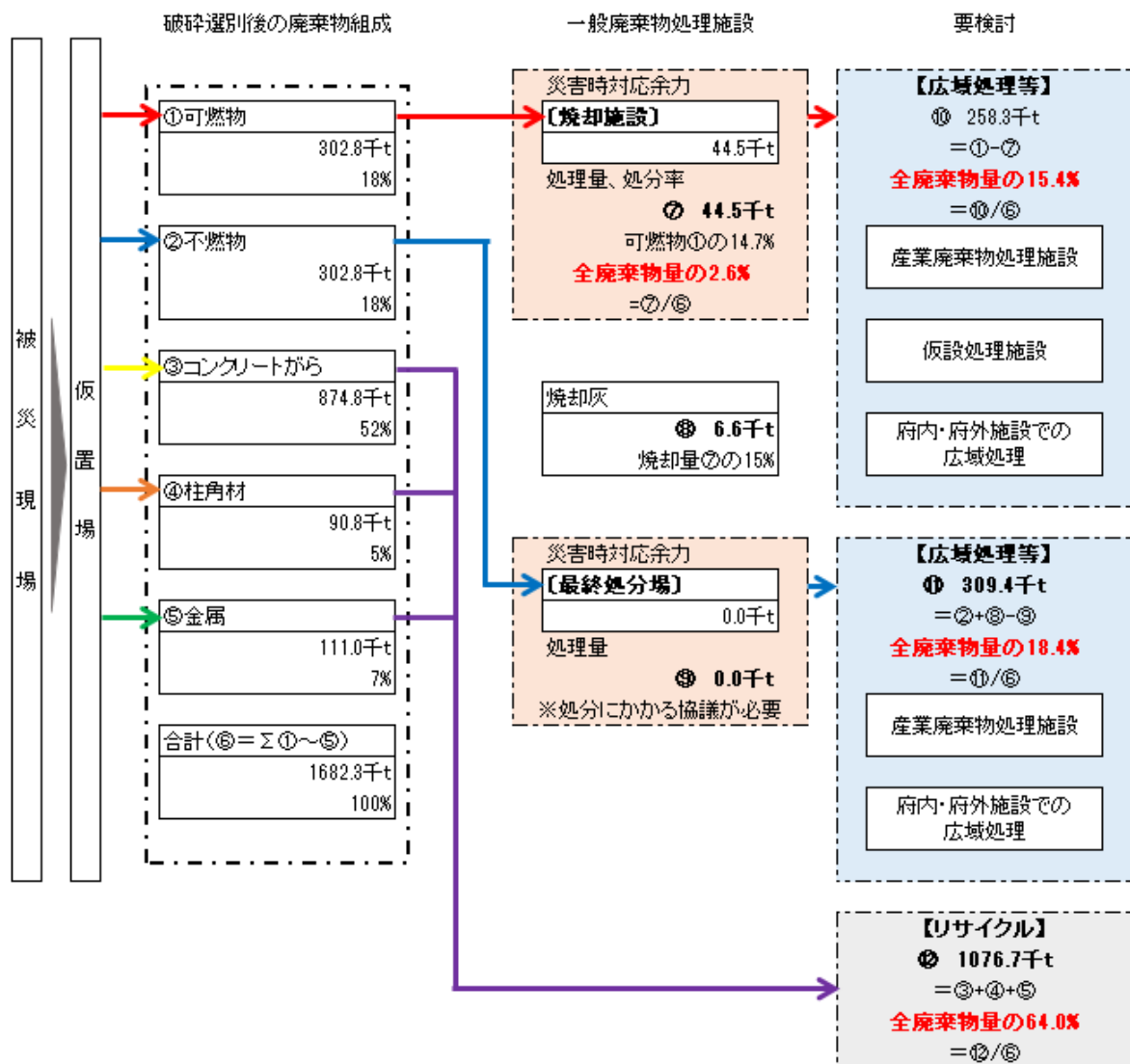
図2-6-2 災害廃棄物処理フロー（地震災害）
