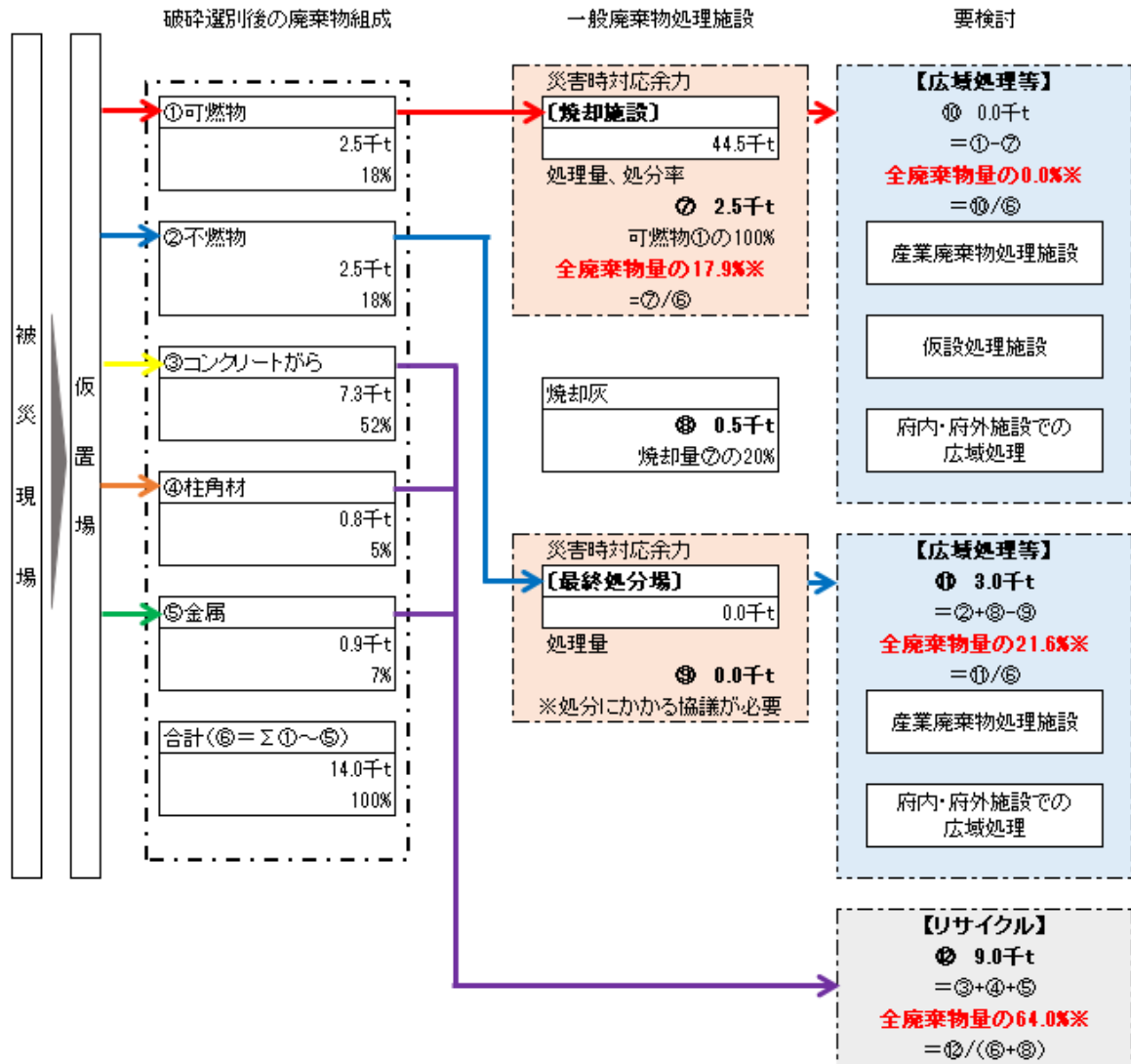
図2-6-3 災害廃棄物処理フロー（風水害）
